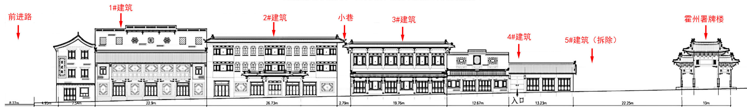
鼓楼东街北侧、霍州署西侧沿街建筑立面改造设计图
